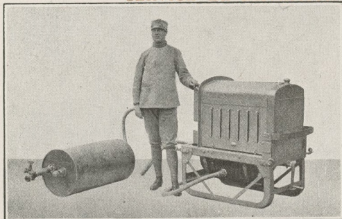
MOTOCOMPRESSEUR DIATTO
